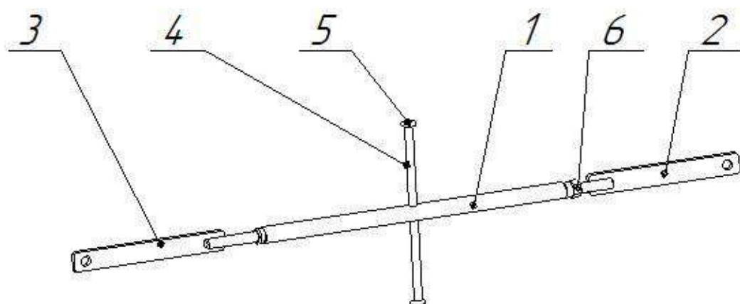
Рис.3 – КСПШ-4.00.100 – Стяжка
